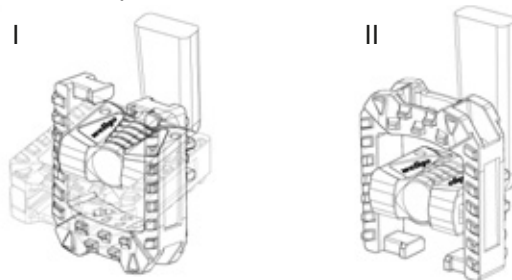
Illustration 84 : Plier la pédale vers le bas (I) ou vers le haut (II)
