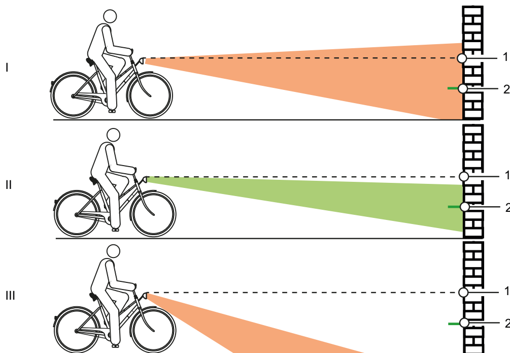
Illustration 71 : Feu réglé trop haut (1), correctement (2) et trop bas (3)
