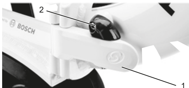
Illustration 88 : Levier de serrage du cadre fermé (1) et levier de blocage du cadre fermé (2)
